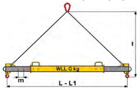
JTPR - Jeřábová traverza pevná (rozpěrná)
