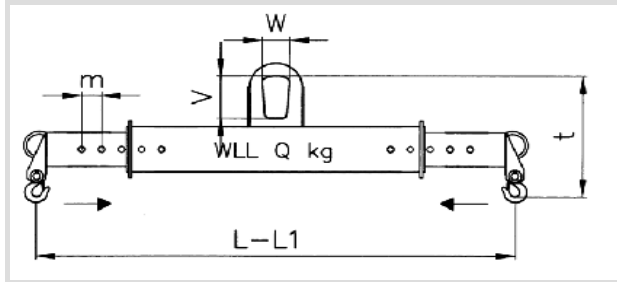
JTS2T - Jeřábová traverza stavitelná - teleskopická
