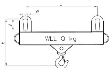
JTP 2J - Jeřábová traverza pevná (dvoujeřábová)
