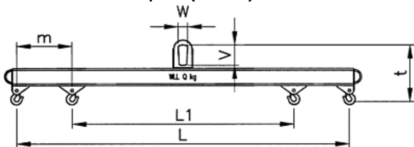
JTPN - Jeřábová traverza pevná (násobná)
