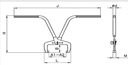
Svěrací kleště na obrubníky Stavitelné
