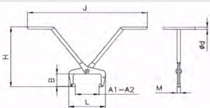
Svěrací kleště na obrubníky
