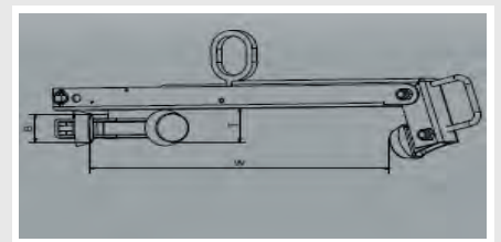
Nosič krycích odpadových vík
